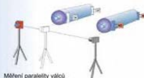
Měření paralelity válců
